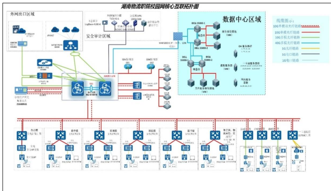
图 6-9 学校数据中心网络拓扑
